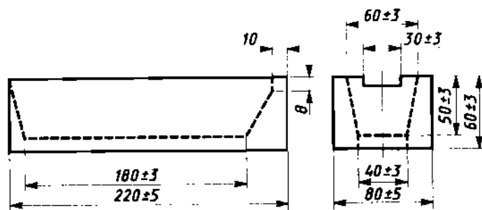
Рисунок 1 — Изложница
